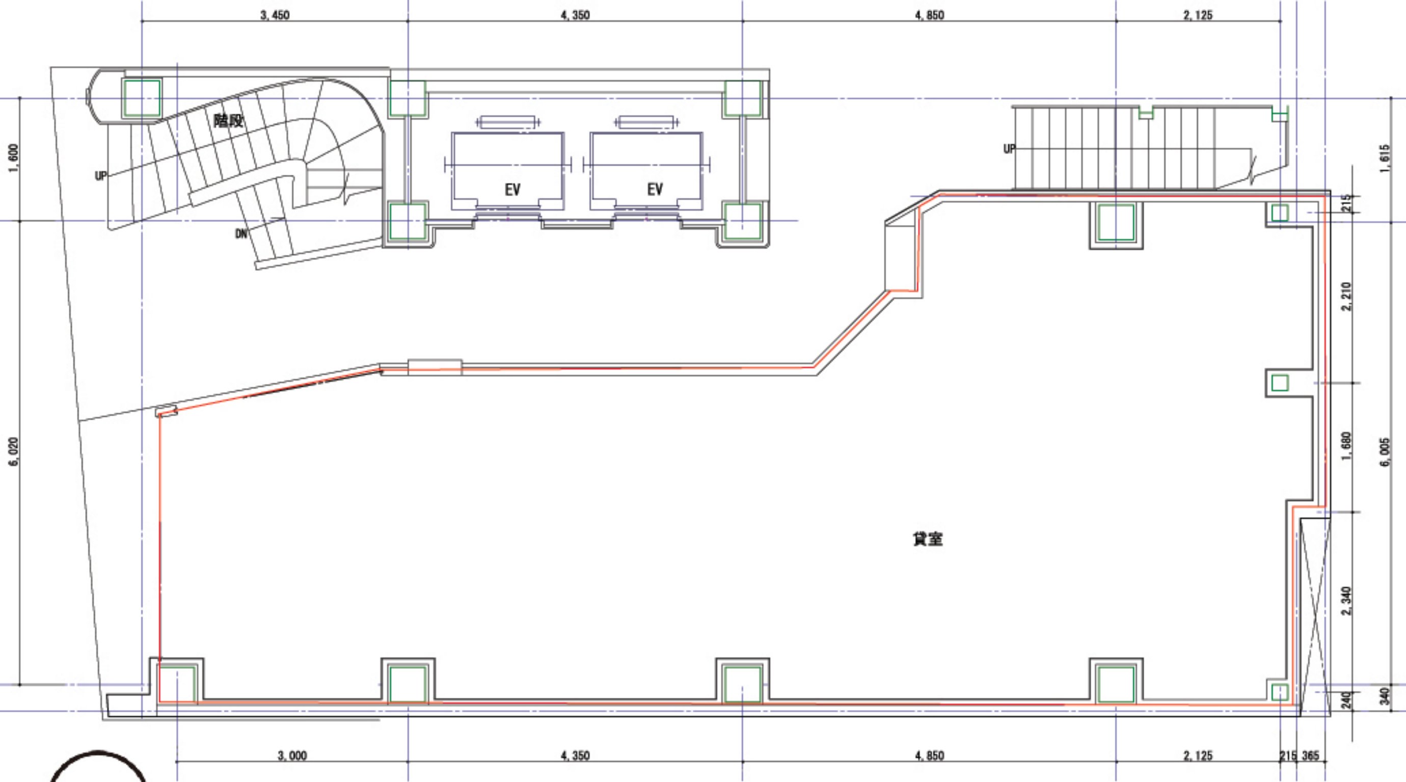
アンテナ21ビル 1階平面図 SCALE 1:50
