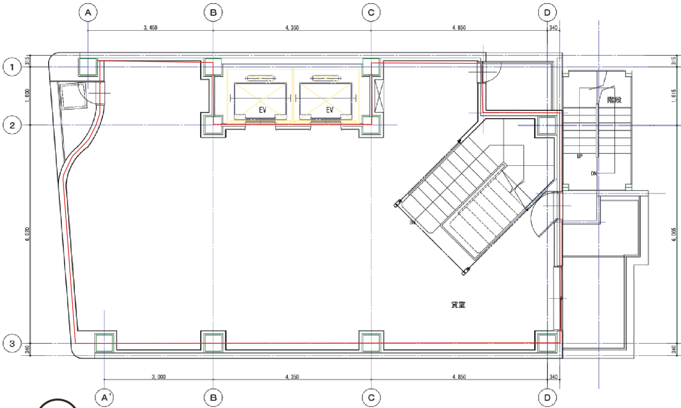
アンテナ21ビル 3階平面図 SCALE 1:50
