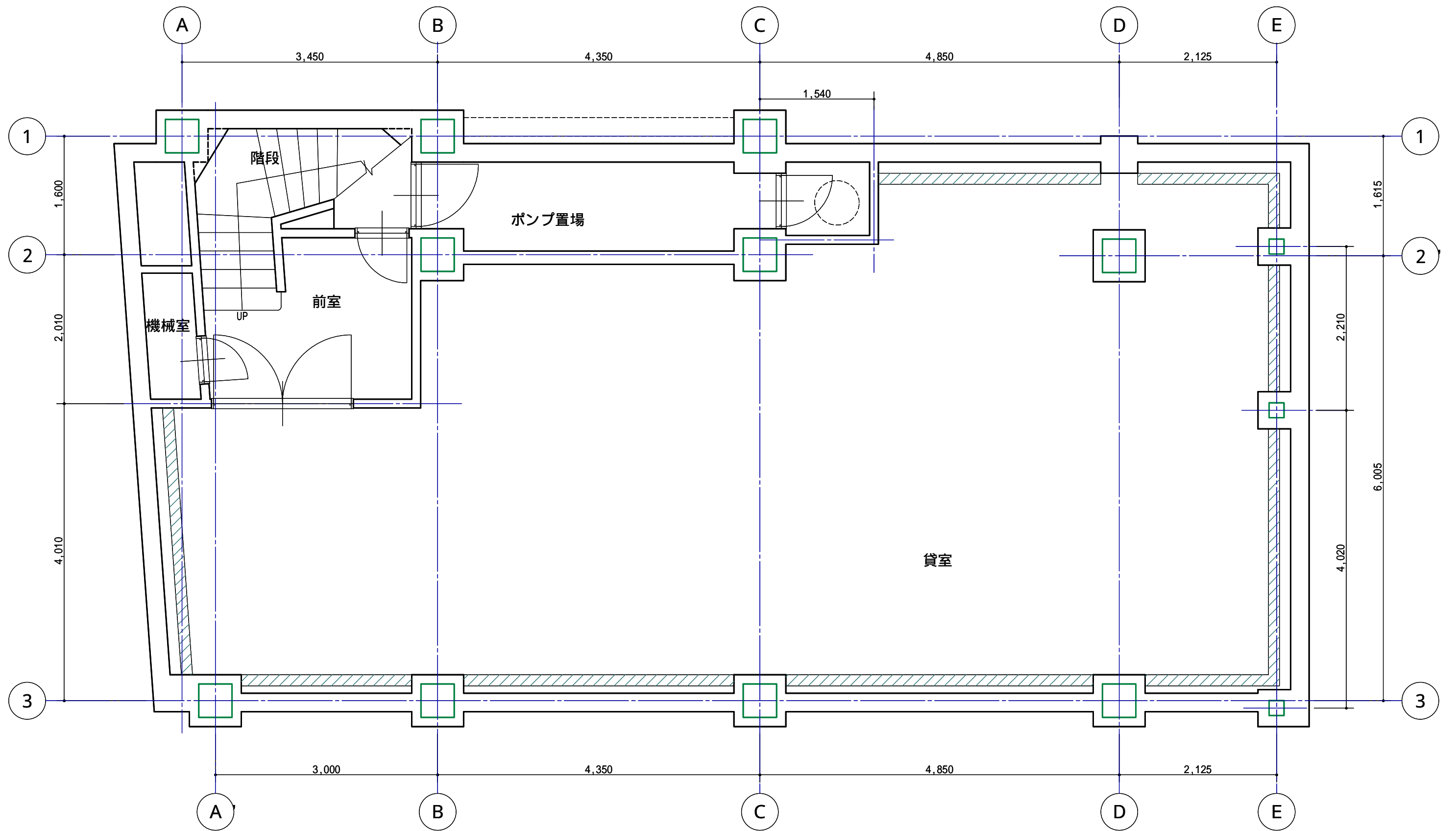
アンテナ21ビル B 1階平面図 SCALE 1:50
